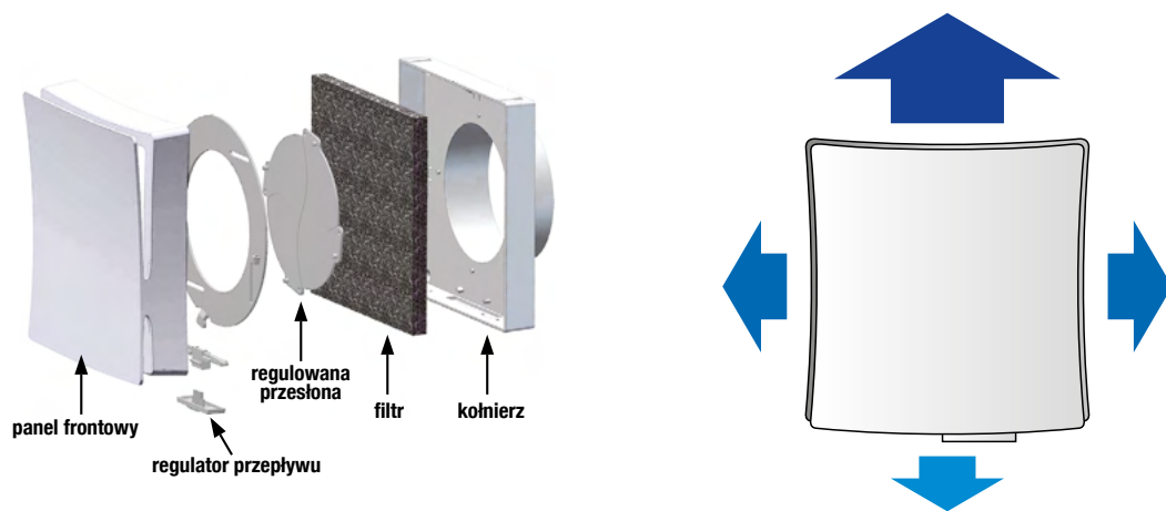
Schemat intensywności rozchodzenia się strumienia nawiewanego powietrza
